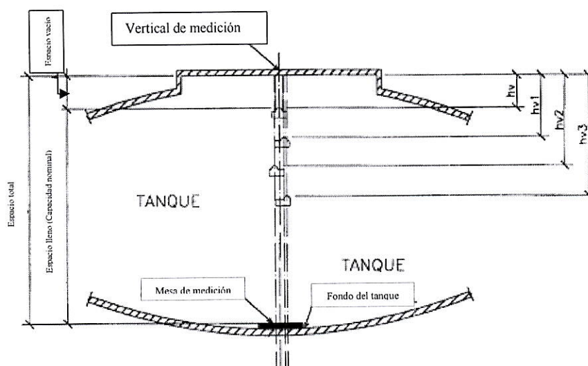
Corte Transversal Esquemático
